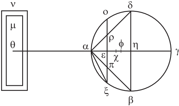
Figura D.2: A figura do Teorema VI na apresentação de E. J. Dijksterhuis.
