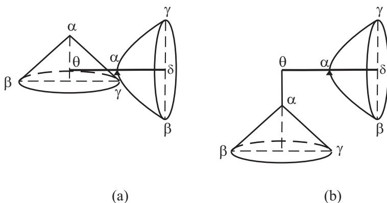
Figura 10.27: (a) Equilíbrio dos sólidos sobre a alavanca ao redor do ponto \alpha com o paraboloide permanecendo em seu lugar distribuído sobre o braço da alavanca, enquanto que o cone está atuando apenas sobre o ponto \theta . (b) Mesma situação de equilíbrio com o cone dependurado em \theta por um fio de peso desprezível, com o paraboloide distribuído sobre o braço da alavanca.
