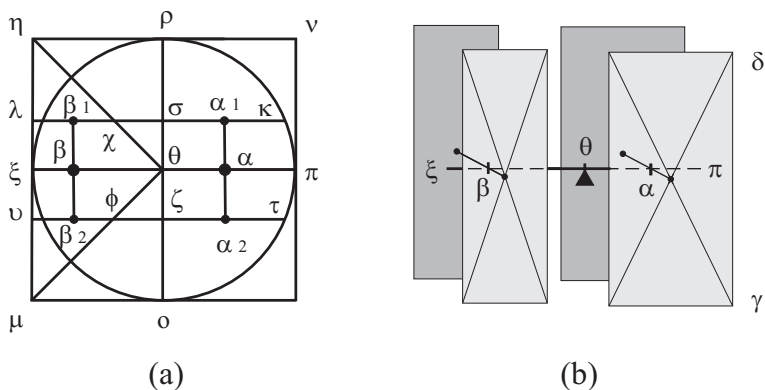
Figura 10.58: (a) Figura considerada por Arquimedes. (b) Visão em perspectiva dos dois paralelogramos do semicilindro passando por οπρ e dos dois paralelogramos do prisma passando por ηθμ .
