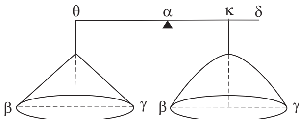
Figura 10.28: Alavanca em equilíbrio ao redor do ponto \alpha com o cone atuando em \theta e o paraboloide atuando em seu centro de gravidade \kappa .
