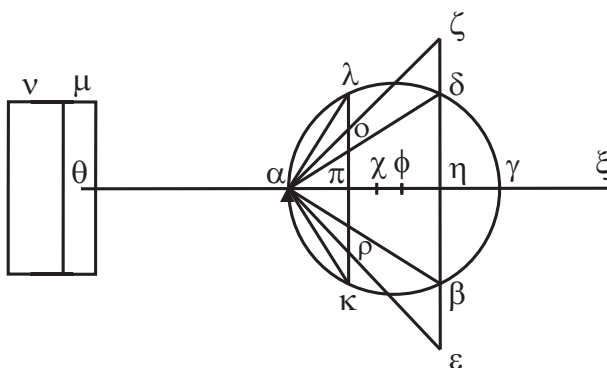
Figura 11.8: Figura do Teorema IX.
