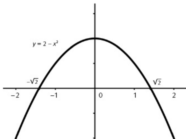
ILUSTRAÇÃO 4 Gráfico da equação y = 2 - x^2 .
