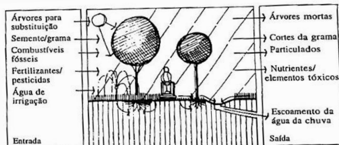
Árvores e gramado Um ecossistema aberto
