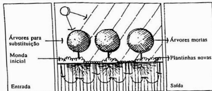
Árvores e cobertura do solo Um ecossistema semifechado
