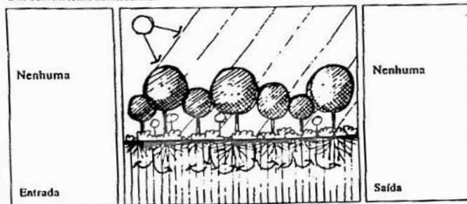
Floresta Um ecossistema fechado
